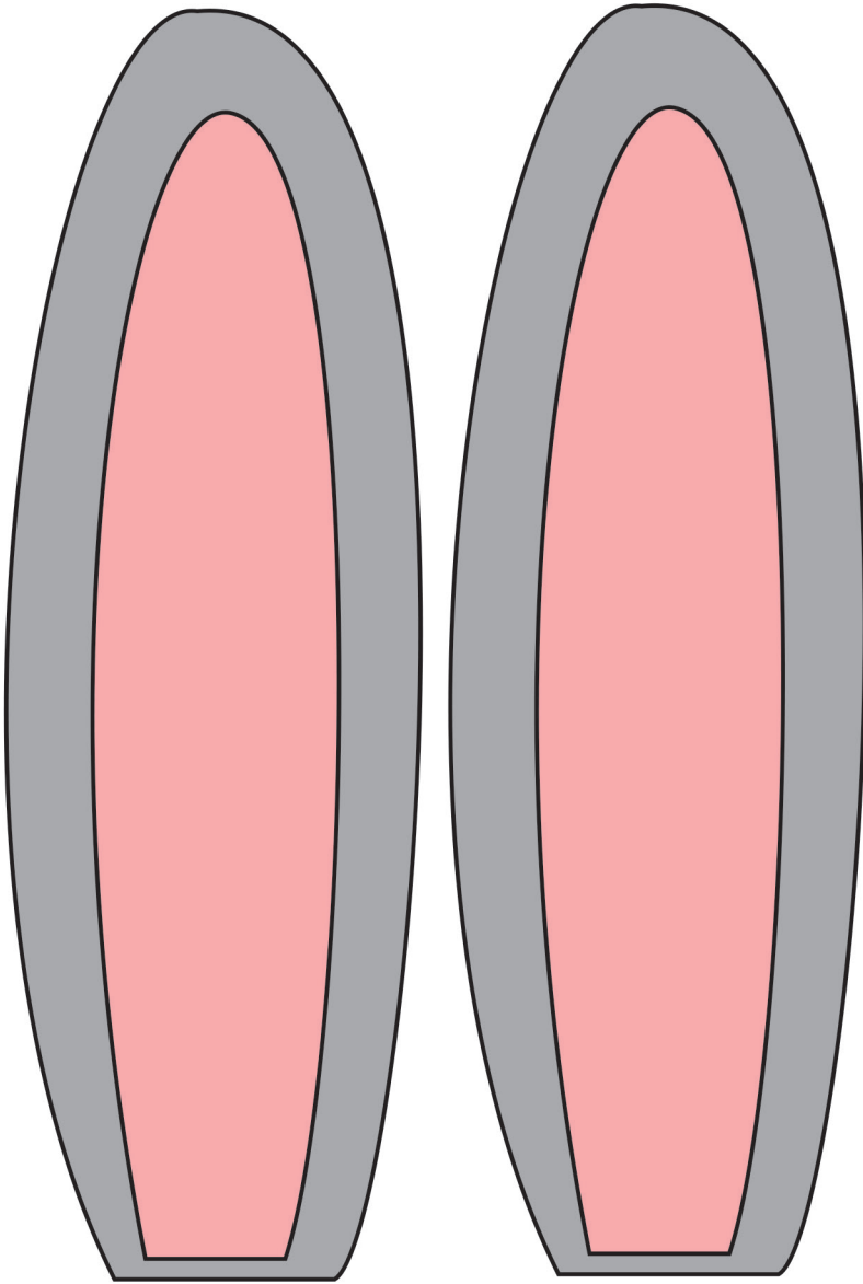
ماسک ۲- گوش‌ها
