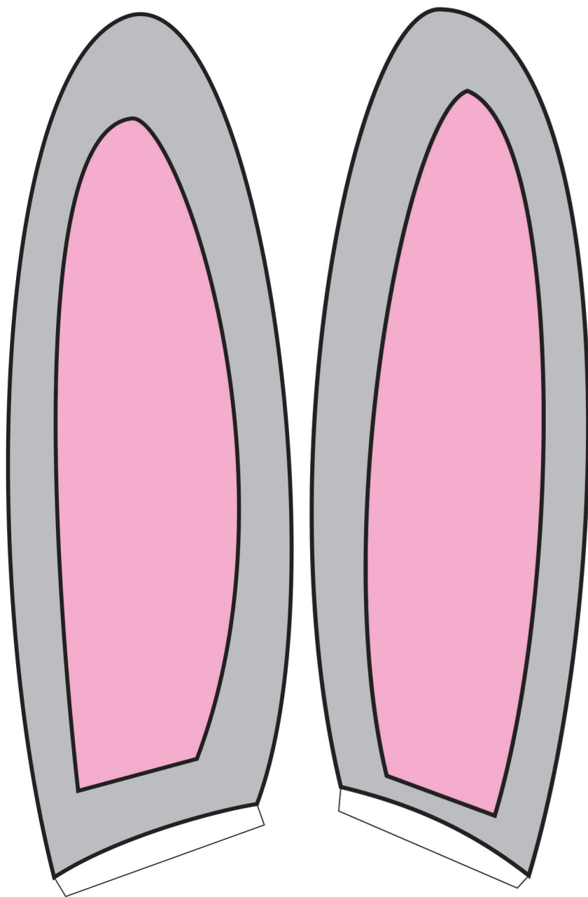
ماسک ۱- گوش‌ها
