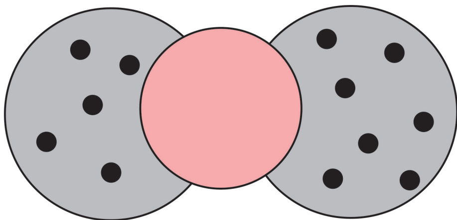
ماسک ۲- بینی
