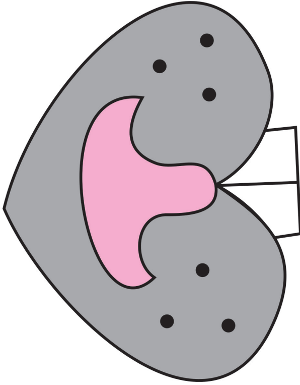
ماسک ۱- شکل ۲
